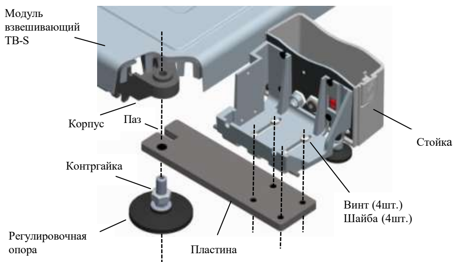
Рис. 2.4 – Крепление терминалов к модулю взвешивающему ТВ
