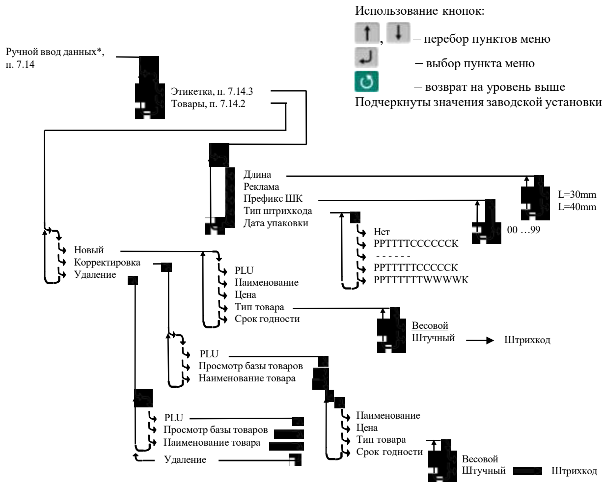
Рис. 7.2 – Схема заполнения справочников с клавиатуры терминала
